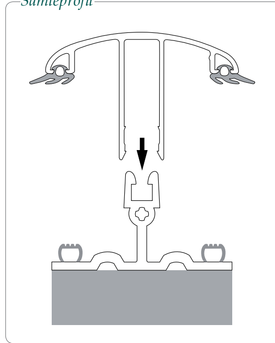
Samleprofil
